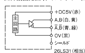
出力段回路図 (ラインドライバ出力形)
