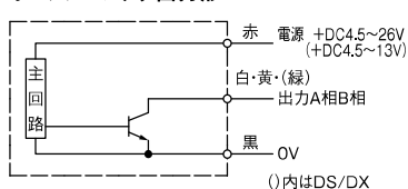
オープンコレクタ出力形
