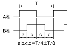
コンプリメンタリ出力形 (電圧出力)
