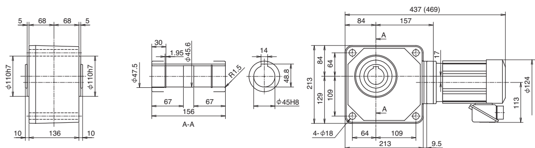
Fig. 5 RNYM05-1530-80~240 Mass 23kg (RNYM05-1530-B-80~240) (Mass 24kg)
