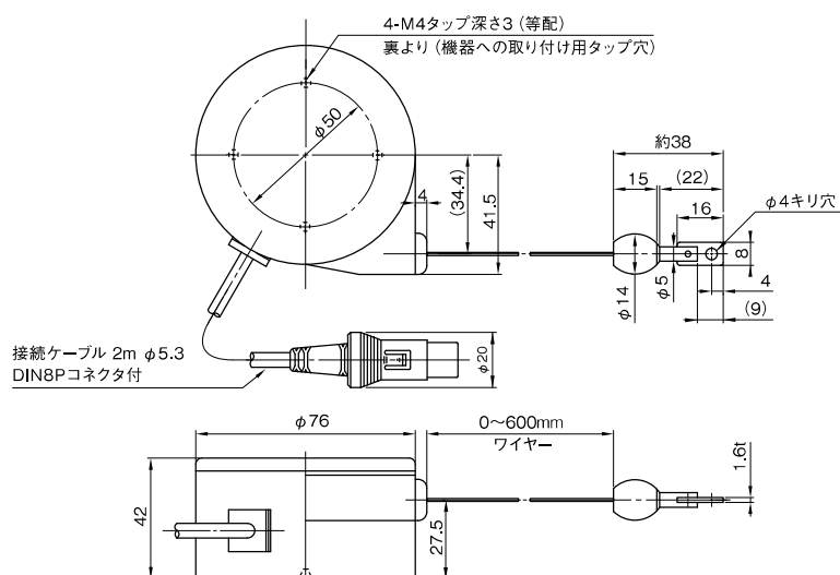
■D-540/D-5400 外形寸法図
