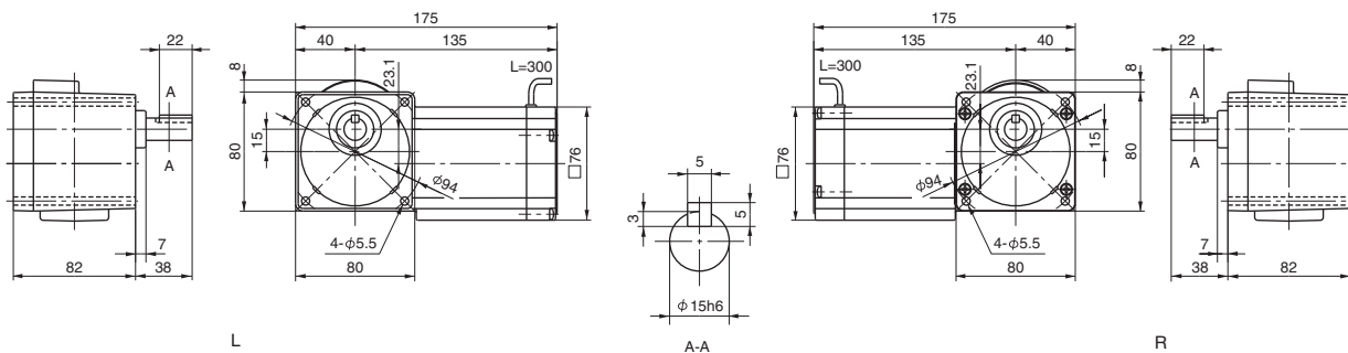
Fig. 2 RNFM0015-03 ½-CC-120-240 Mass 2.7kg
