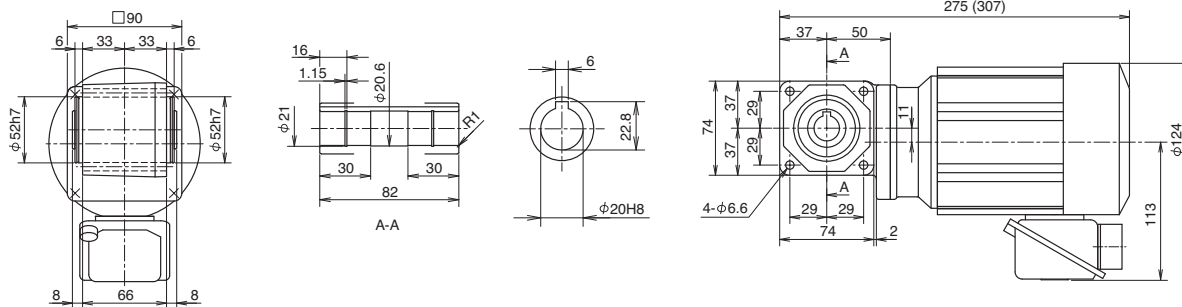
Mass 7.0kg (Mass 8.5kg)
