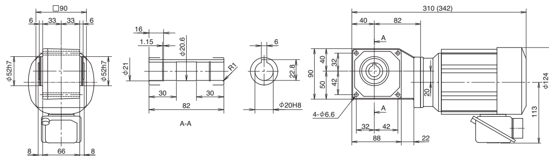
Mass 7.0kg (Mass 8.5kg)
