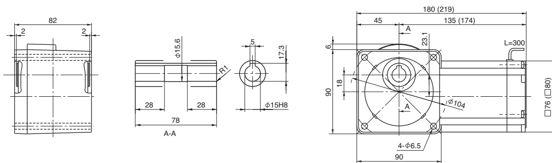
Fig. 2 RNYM004-17-150~240 (RNYM004-17-B-150~240) Mass 3.7kg (Mass 4.1kg)
